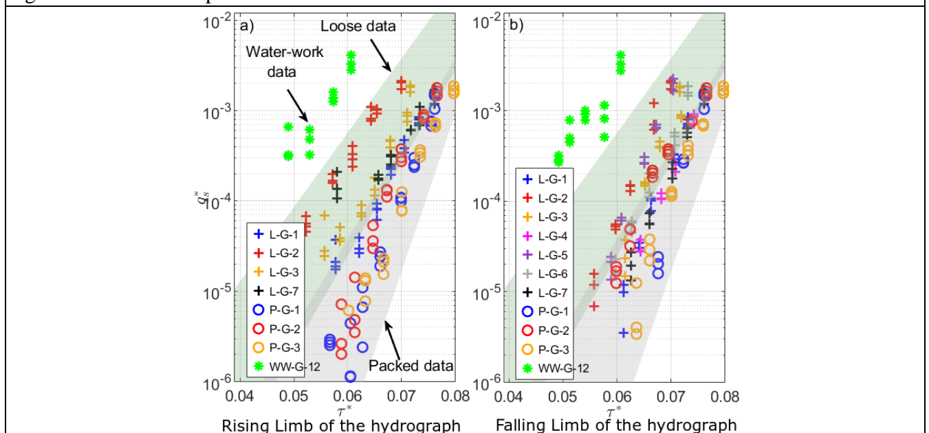
Figure 2 – Impact de l'arrangement du lit sur le transport solide (L : loose bed, P : packed bed, WW : water-worked bed)
